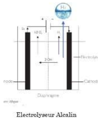
Schéma d'un électrolyseur alcalin
